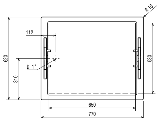
Boven aanzicht
